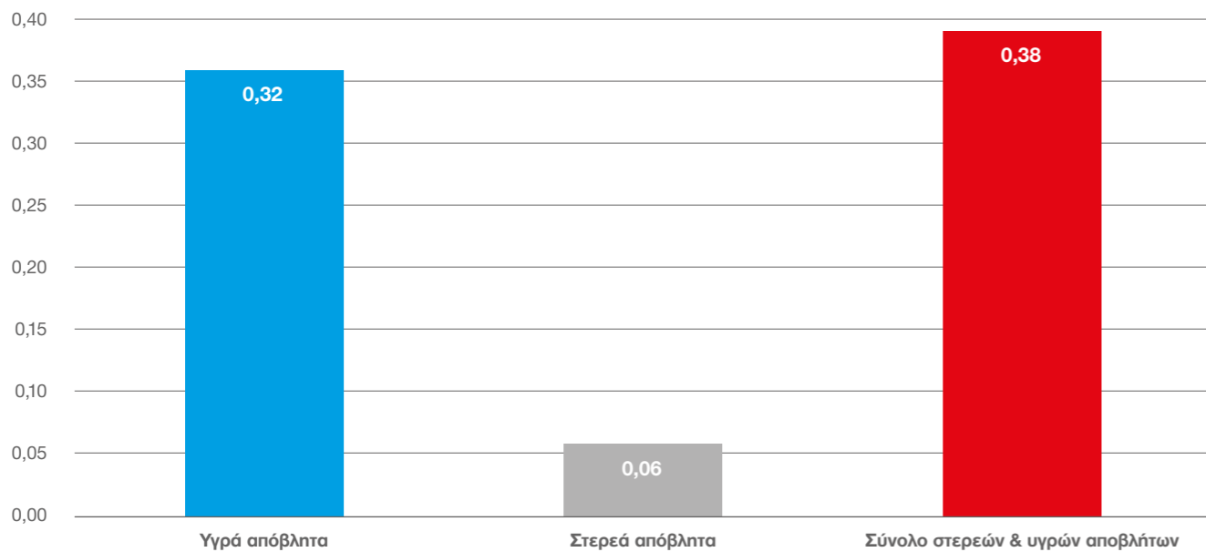
Ένταση παραγόμενων υγρών και στερεών αποβλήτων (tn αποβλήτων/tn παραγόμενου προϊόντος) στο εργοστάσιο Ασπροπύργου, το 2024
