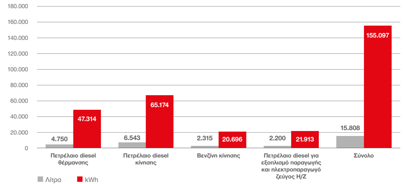
Κατανάλωση Ορυκτών Καυσίμων (kWh) Εργοστασίου Ασπροπύργου 2024
